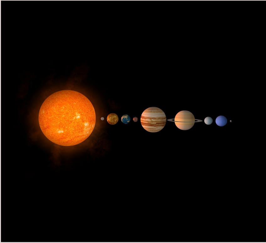
Système Solaire
